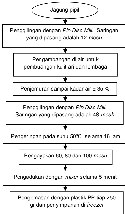
Gambar 1. Proses pembuatan tepung jagung
