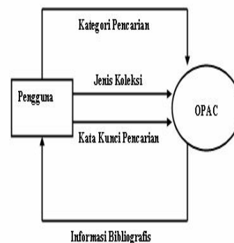
Gambar 1 Diagram Konteks
