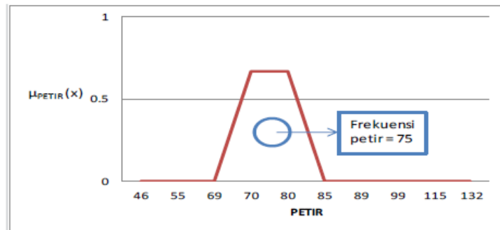
Gambar 8 Hasil Perhitungan dari Agregasi Semua Aturan Model Frekuensi Petir
